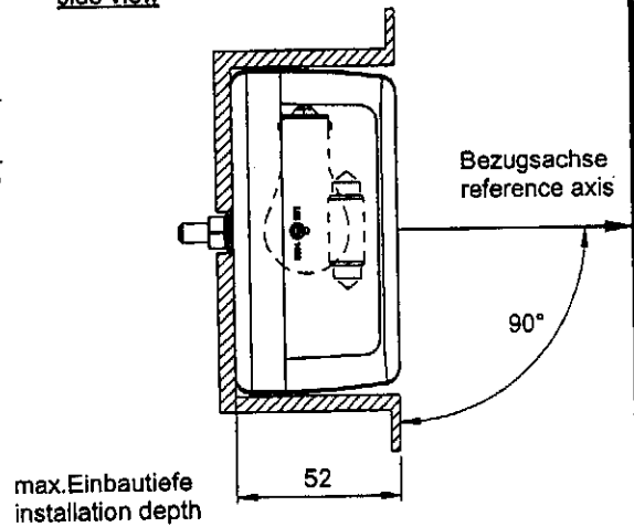
Ansicht von der Seite/ side view
