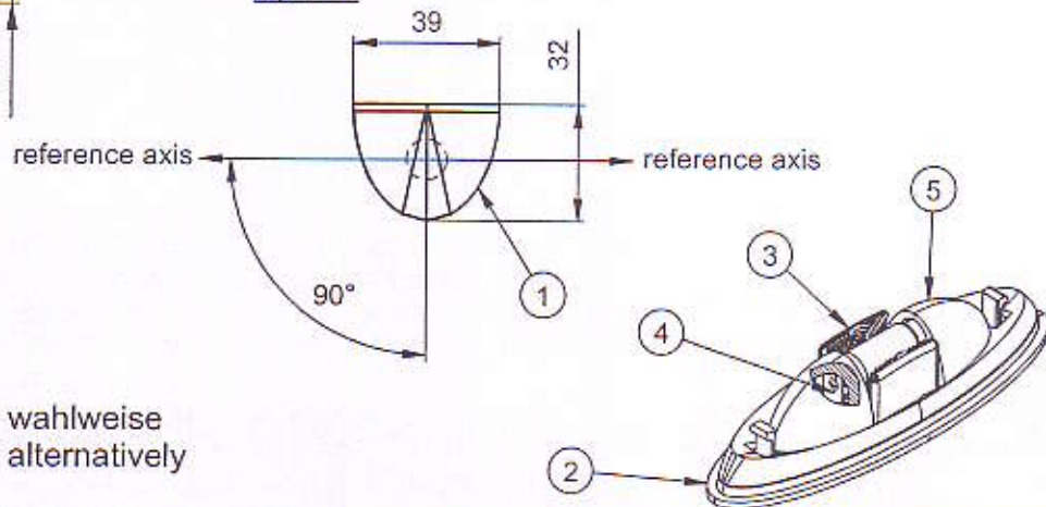
Ansicht von Oben / top view
