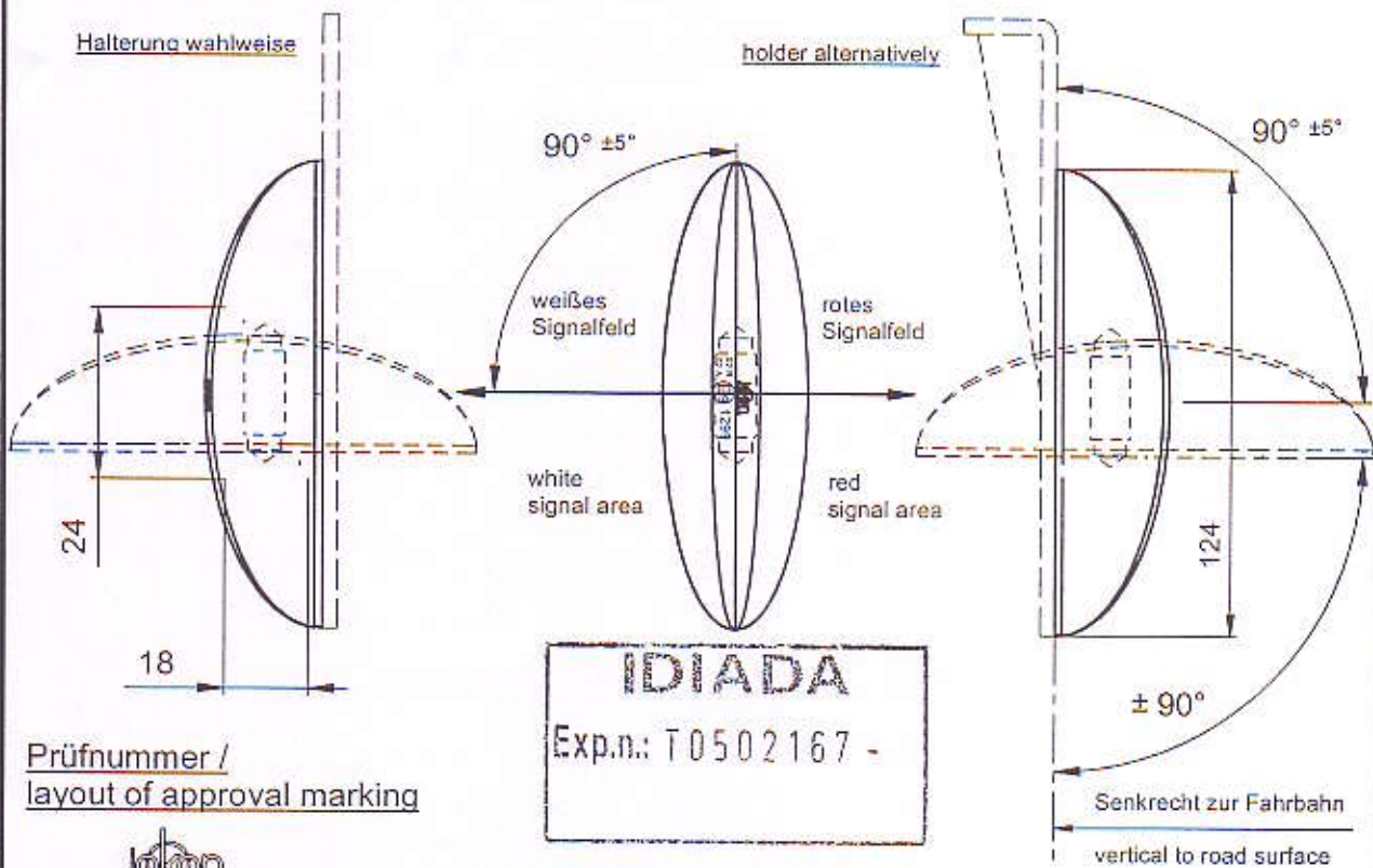
Ansicht von Oben / top view
