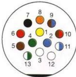
Bilden visar kontakt på dragbil
