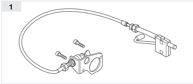
Mechanische Fernbedienung (40, 50 mm) (RC-MS) • Mechanical remote control (40, 50 mm) (RC-MS) • Commande à distance mécanique (40, 50 mm) (RC-MS) • Apertura meccanica a distanza (40, 50 mm) (RC-MS) • Telemando mecánico (40, 50 mm) (RC-MS)
