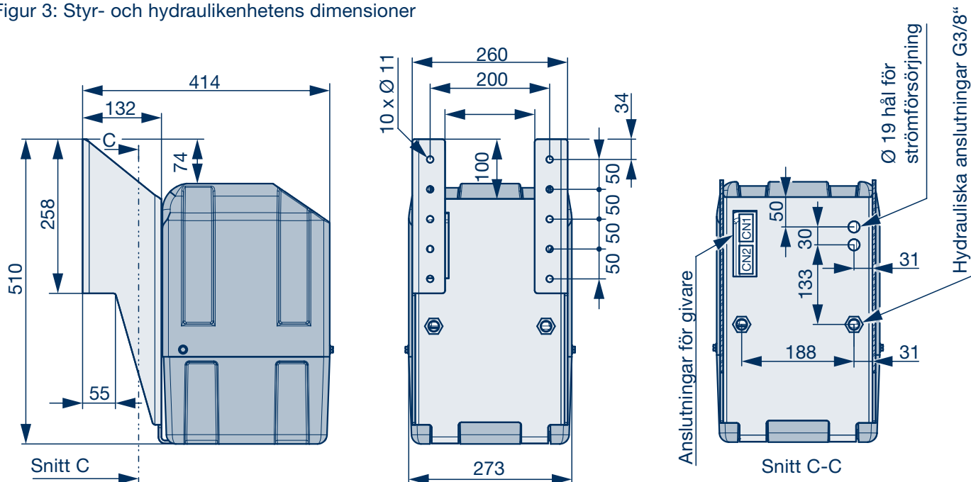
Figur 3: Styr- och hydraulikenhetens dimensioner
