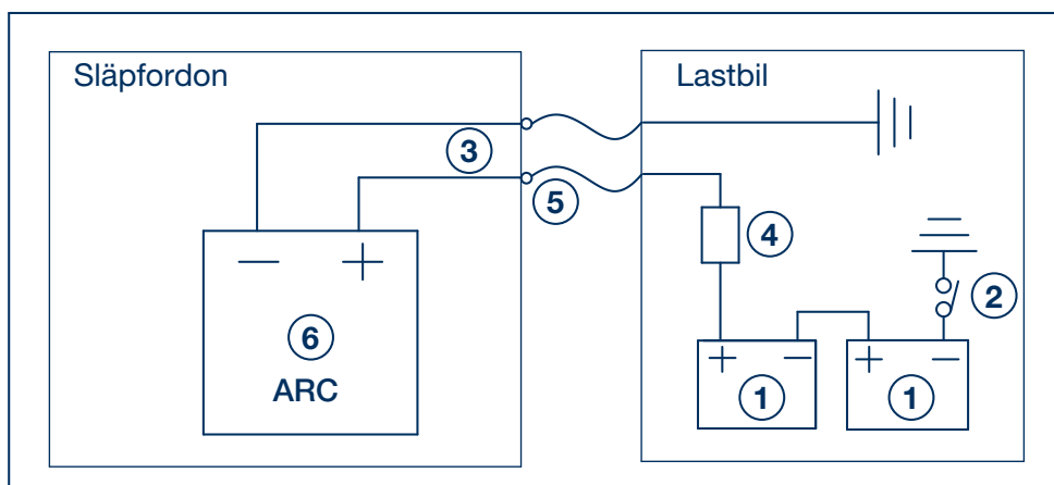
Exempel 2. Negativt chassi, negativt tändlås
