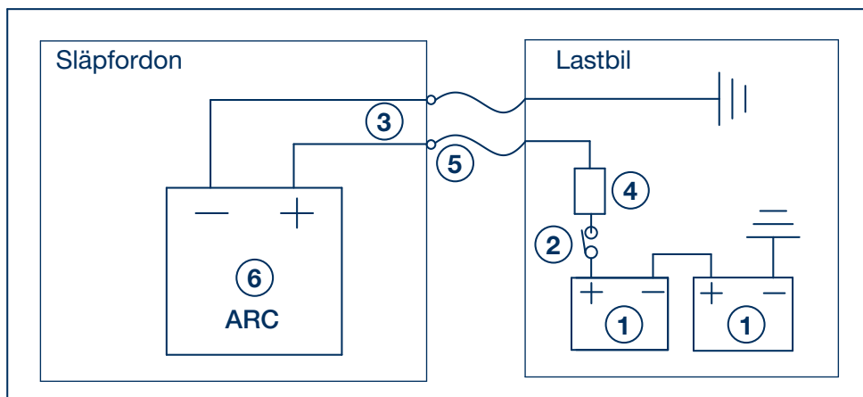
Exempel 1. Negativt chassi, positivt tändlås
